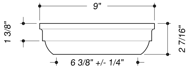
Cap
